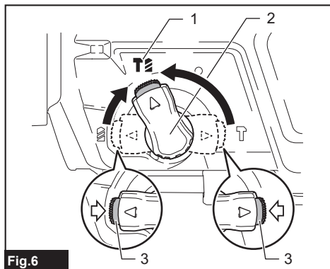
Fig.6 ► 1. Rotation avec percussion 2. Bouton de changement de mode 3. Bouton de libération
